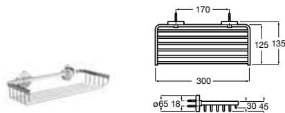
Jabonera ducha
