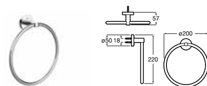
Toallero anilla
