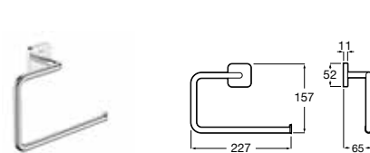
Toallero anilla
