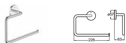
Toallero anilla
