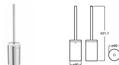
Escobillero suelo
