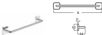
Toallero
