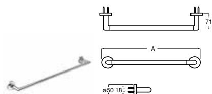
Toallero
