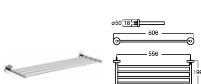
Toallero estante
