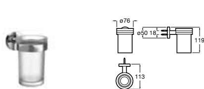
Portacepillos pared
