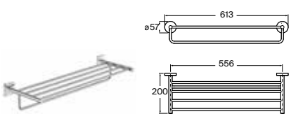
Toallero estante*
