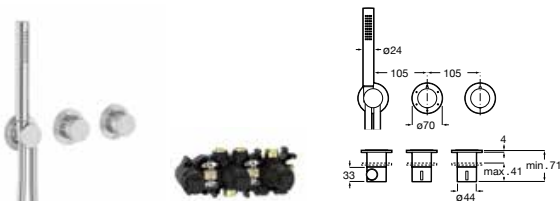
Grifería termostática empotrable 3 vías con ducha de mano y soporte con toma de agua
