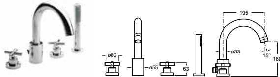
Grifería de repisa para baño-ducha Con caño central alto con inversor, ducha de mano y flexible de 1,75 m Cromado A5A0943C00
