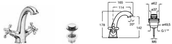
Grifería para lavabo con cuerpo liso Con aireador, desagüe click-clack y enlaces de alimentación flexibles Cromado A5A3A4BC00
