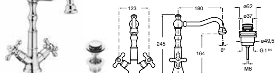
Grifería para lavabo con caño alto y cuerpo liso Con caño alto giratorio, aireador, desagüe click-clack y enlaces de alimentación flexibles Cromado A5A384BC00
