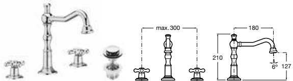
Grifería para lavabo con cuerpo liso Con caño central giratorio, aireador, desagüe click-clack y enlaces de alimentación flexibles Cromado A5A444BC00
