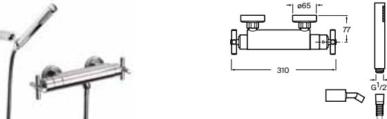
Grifería termostática exterior para ducha Con ducha de mano, flexible de 1,50 m y soporte articulado Cromado A5A1343C00
