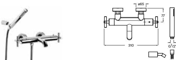
Grifería termostática exterior para baño-ducha Con inversor automático, ducha de mano, flexible de 1,70 m y soporte articulado Cromado A5A1143C00
