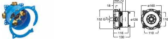
RocaBox Universal Rocabox Universal A525869403 Kit prolongación interna (20 mm) A525564303 Kit florón Round de alargó (20 mm) A525564600 Kit florón Square de alargó (20 mm) A525564700
