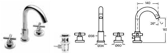
Grifería para lavabo Con caño central giratorio, aireador, desagüe automático y enlaces de alimentación flexibles Cromado A5A4443C00
