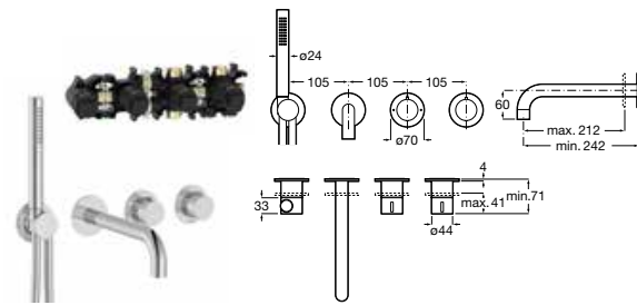
Grifería termostática empotrable 2 vías con ducha de mano, soporte con toma de agua y caño de bañera
