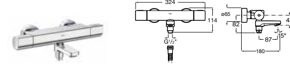
Grifería termostática exterior para baño- ducha Con inversor automático
