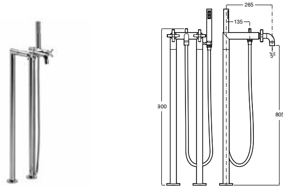
Grifería bimando de pie para baño-ducha Con inversor automático, ducha de mano, flexible de 1,75 m, soporte articulado y columnas verticales de alimentación Cromado A5A2743C00
