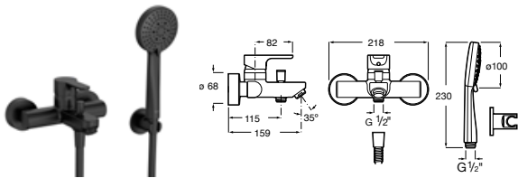
Grifería exterior para baño-ducha Con inversor automático con retención, ducha de mano Stella 100/3F, flexible 1,75m PVC satinado y soporte fijo Negro mate A5A0109NB4
