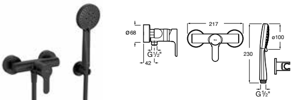
Grifería exterior para ducha Con ducha de mano Stella 100/3F, flexible 1,75m PVC satinado y soporte fijo Negro mate A5A2009NB4
